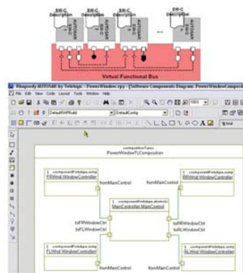
Среда разработки Rhapsody позволяет создавать AUTOSAR-системы, используя термины и нотации, привычные автомобильным инженерам
